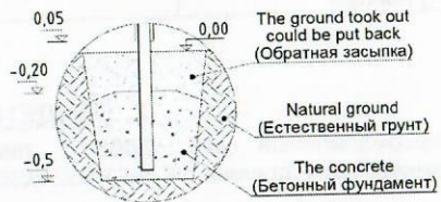
The equipment mounting plan (Схема монтажа оборудования)
